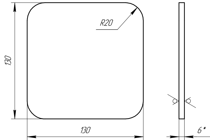
Дет. поз. 2
