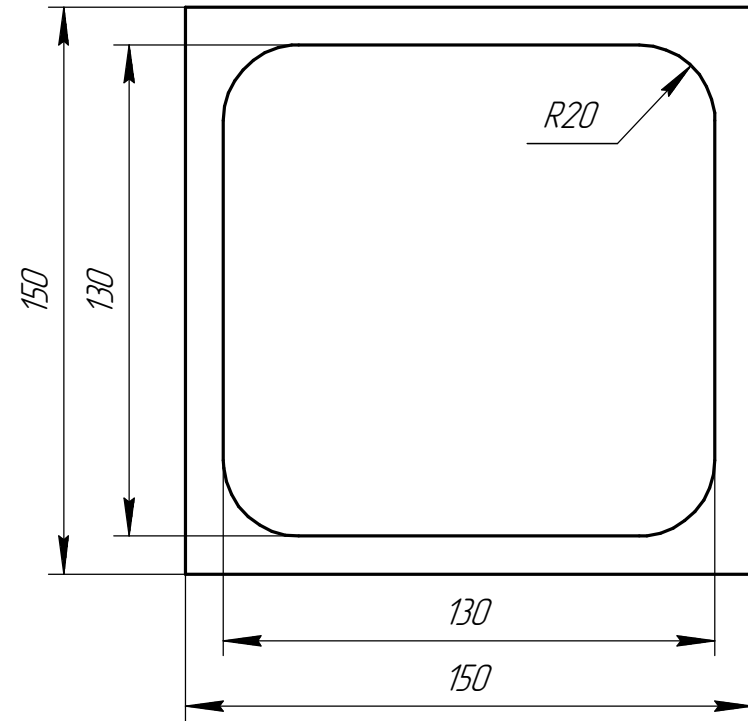
Дет. поз. 1
